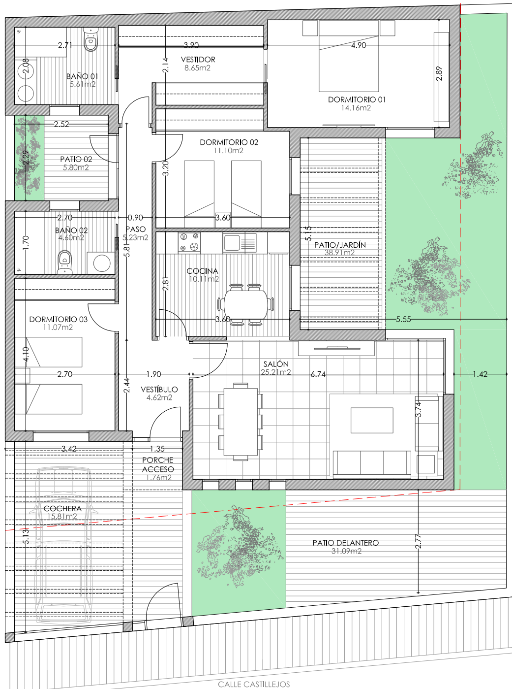
PLANTA BAJA
