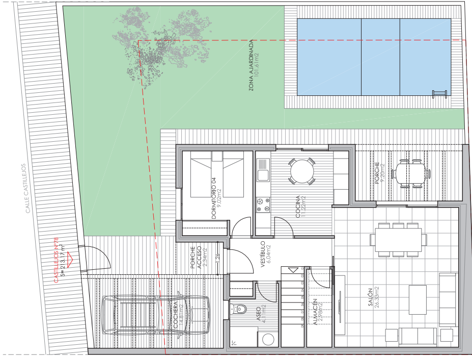
PLANTA BAJA
