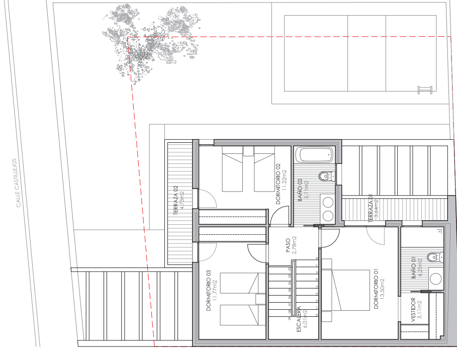
PLANTA PRIMERA
