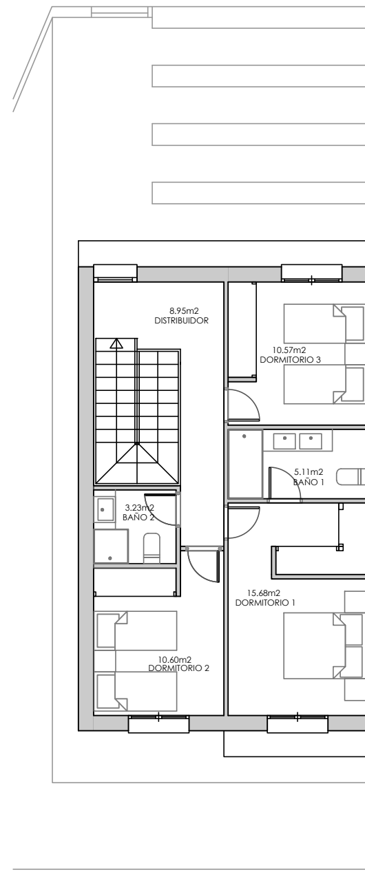
PLANTA 1
