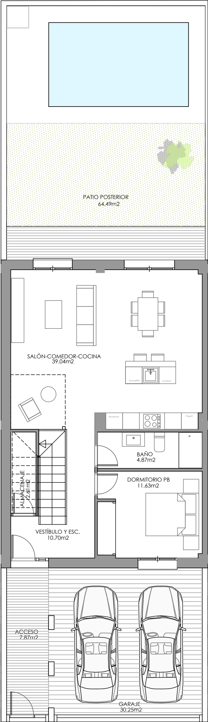
PLANTA BAJA
