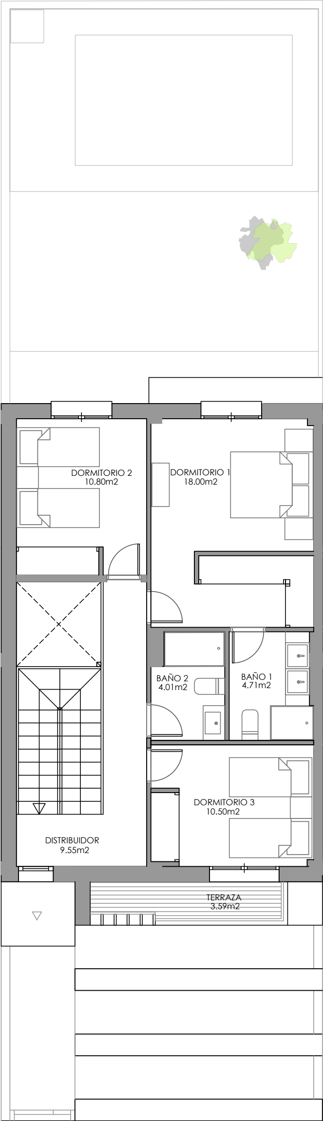
PLANTA 1
