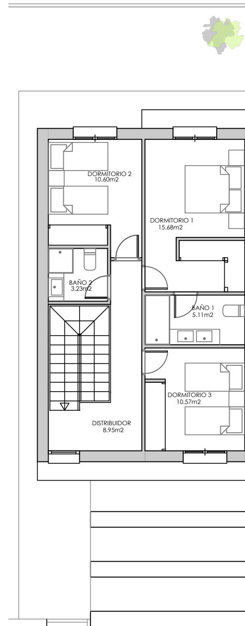
PLANTA 1
