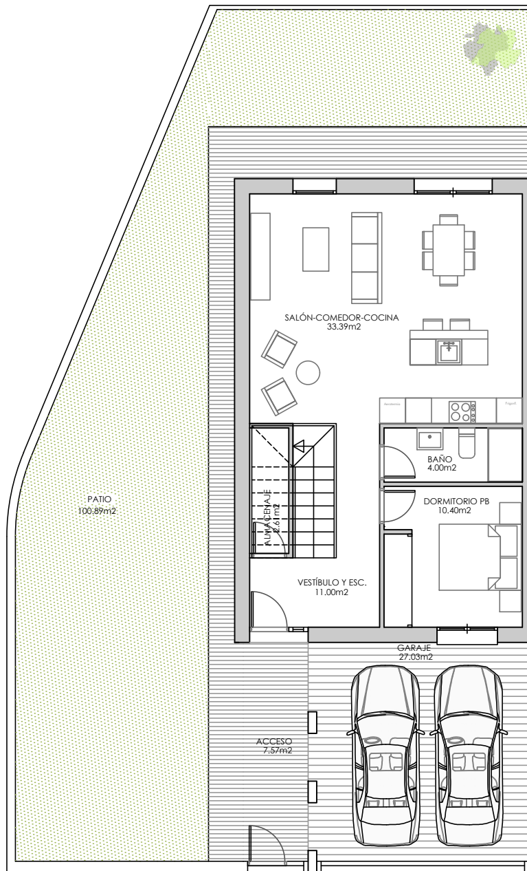
PLANTA BAJA
