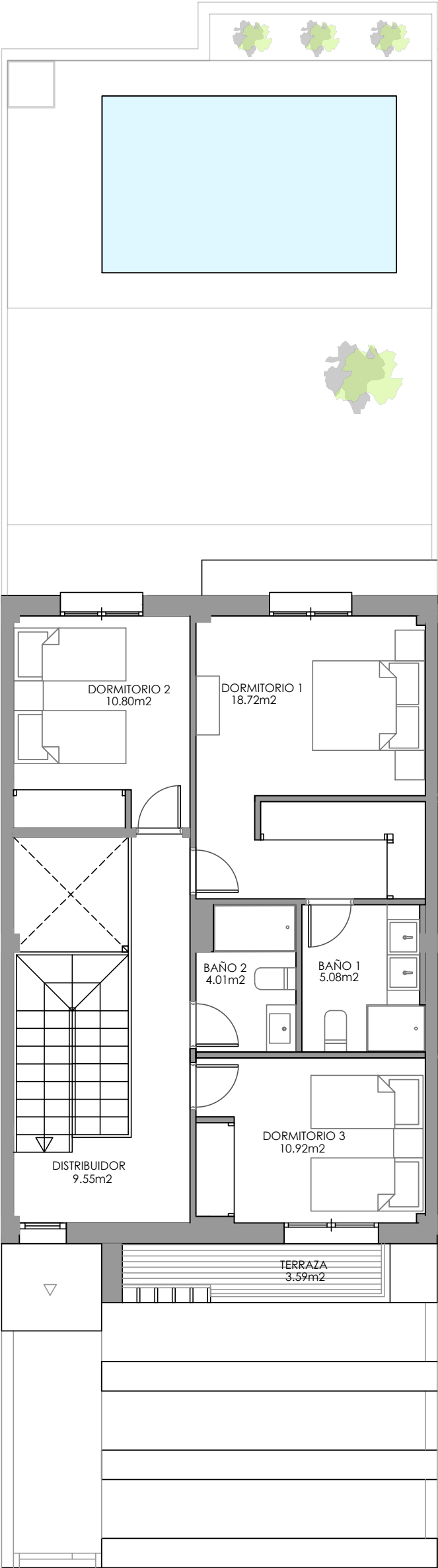
PLANTA 1
