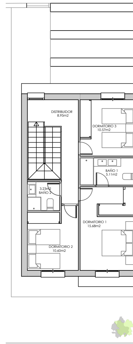
PLANTA 1
