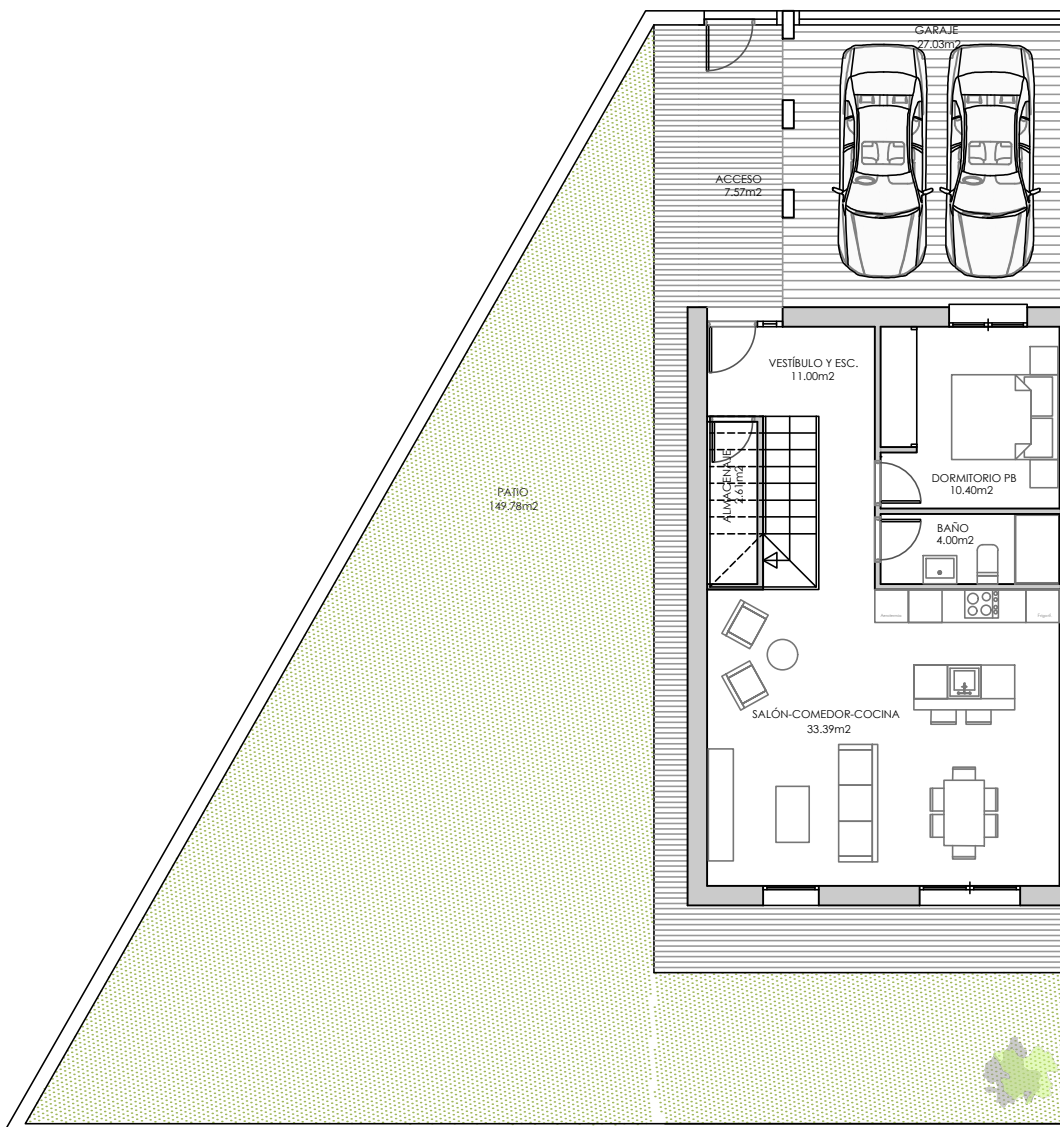
PLANTA BAJA
