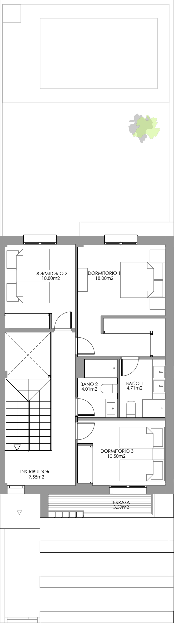
PLANTA 1
